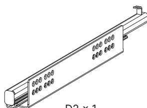
D2 × 1 Skuffeskinne R - Drawer sliders R (1 styk)
